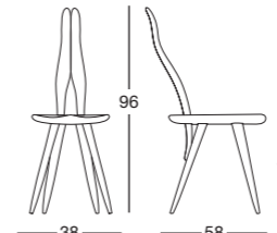
2051 Fenis CM Carlo Mollino, 1959
